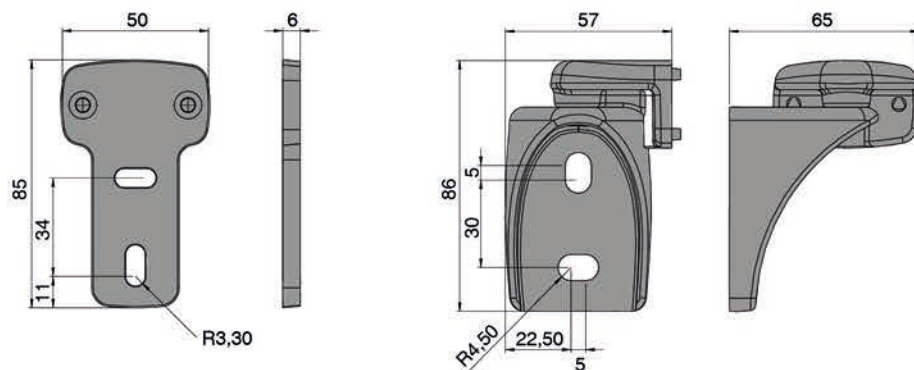
Fixation entre tableau
