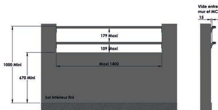
MODY 1 lisse en applique
