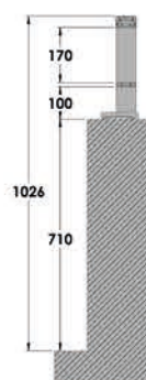
Sur Muret avec 1 lisse
