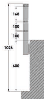
Sur Muret avec 2 lisses
