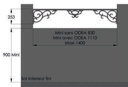
LISEA entre tableau
